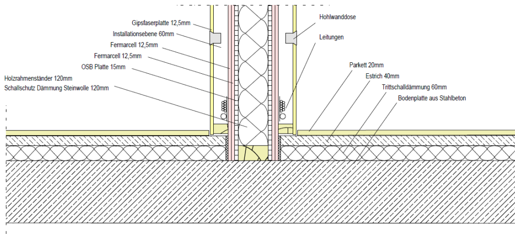
Abbildung 8: Erdgeschoss, Trennwände
